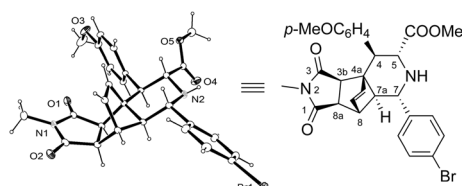
Figure 1. X-ray structure of (3 a R ,3 b S ,4 R ,5 R ,7 S ,7 a S ,8 R ,8 a R )- 11d .
